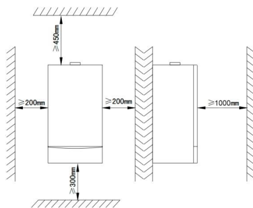
Рис. 11.1. Размещение котла
